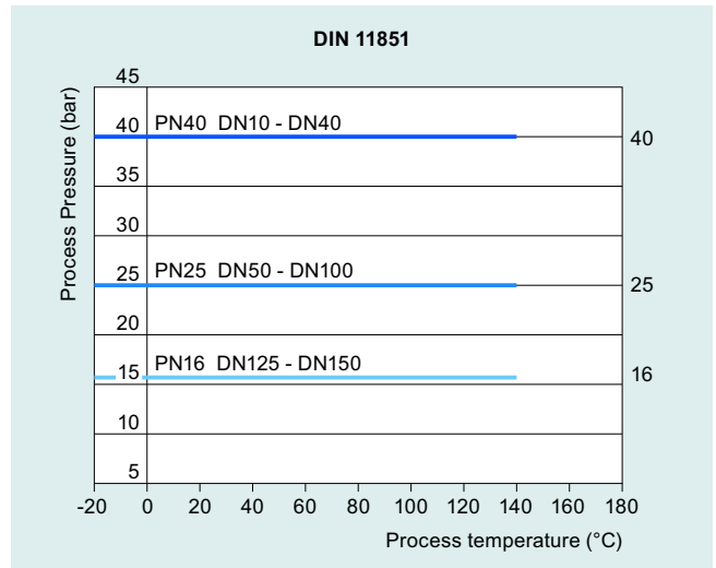
DIN 11581 flanges stainless steel (PN 25 ... PN 40)
